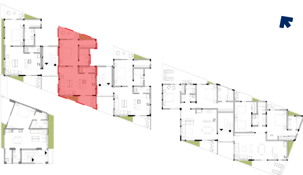
SEGUNDO NIVEL
