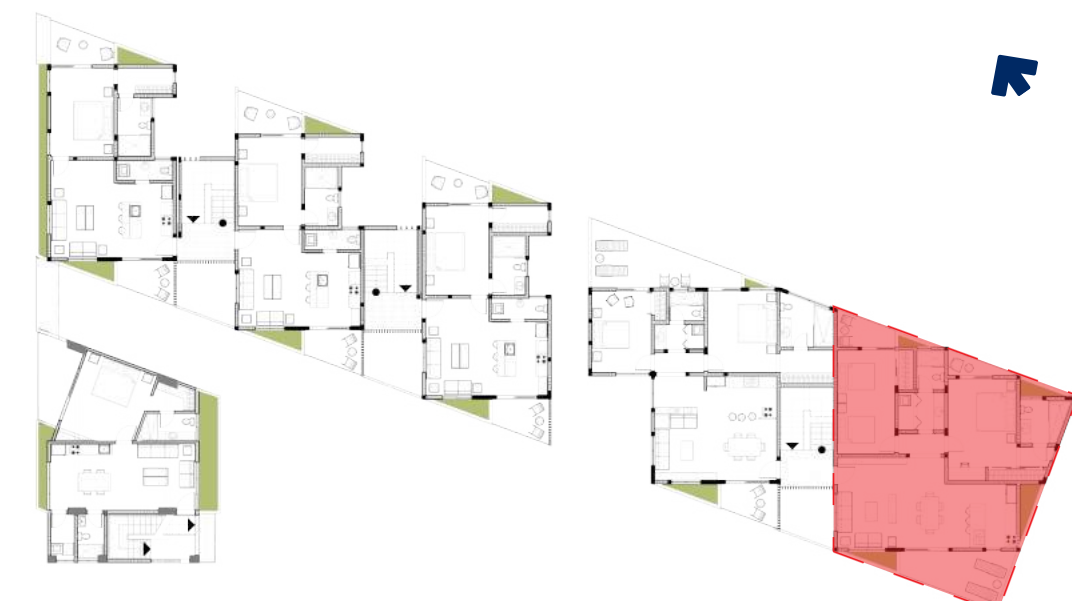
SEGUNDO NIVEL
